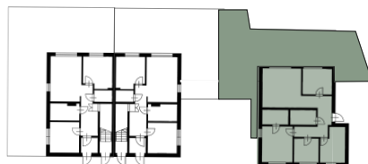
Układ budynków
